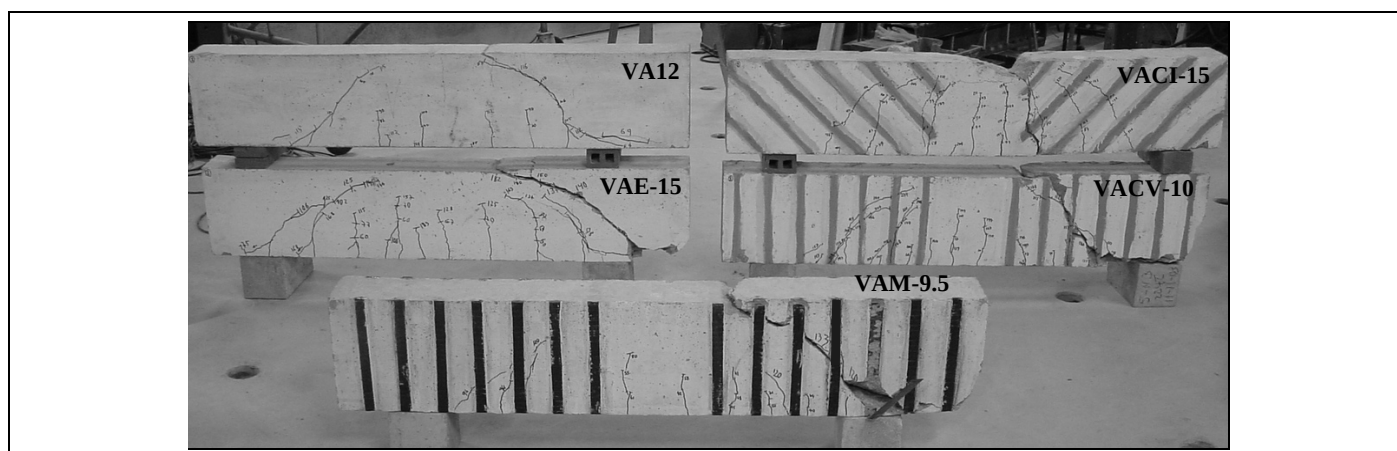
Figura 10 - Modos de rotura das vigas da série A com 4φ12 longitudinais.
