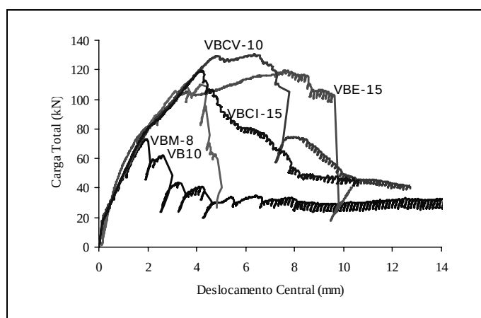
Figura 11 - Curvas carga total vs deslocamento central das vigas da série B com 4φ10 longitudinais.
