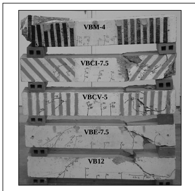
Figura 14 - Modos de ruína das vigas da série B com 4 \phi 12 longitudinais.
