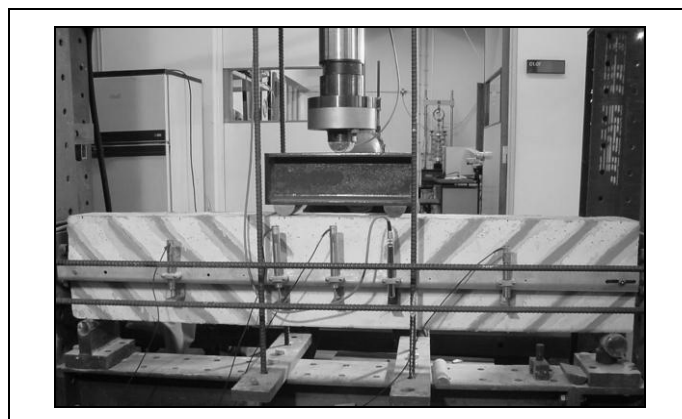
Figura 5 - Esquema geral do ensaio das vigas.
