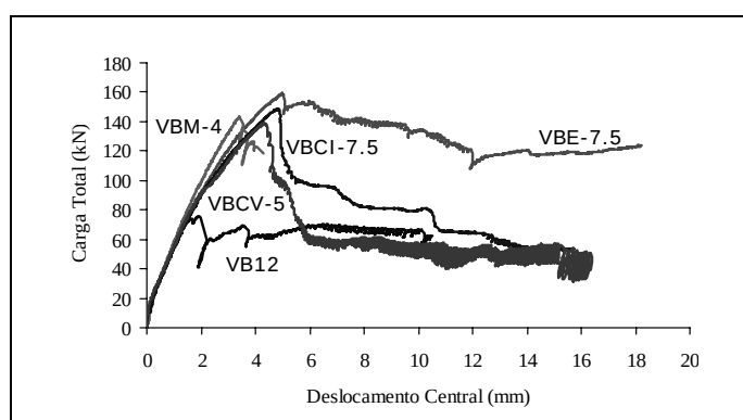
Figura 13 - Curvas carga total vs deslocamento central das vigas da série B com 4 \phi 12 longitudinais.
