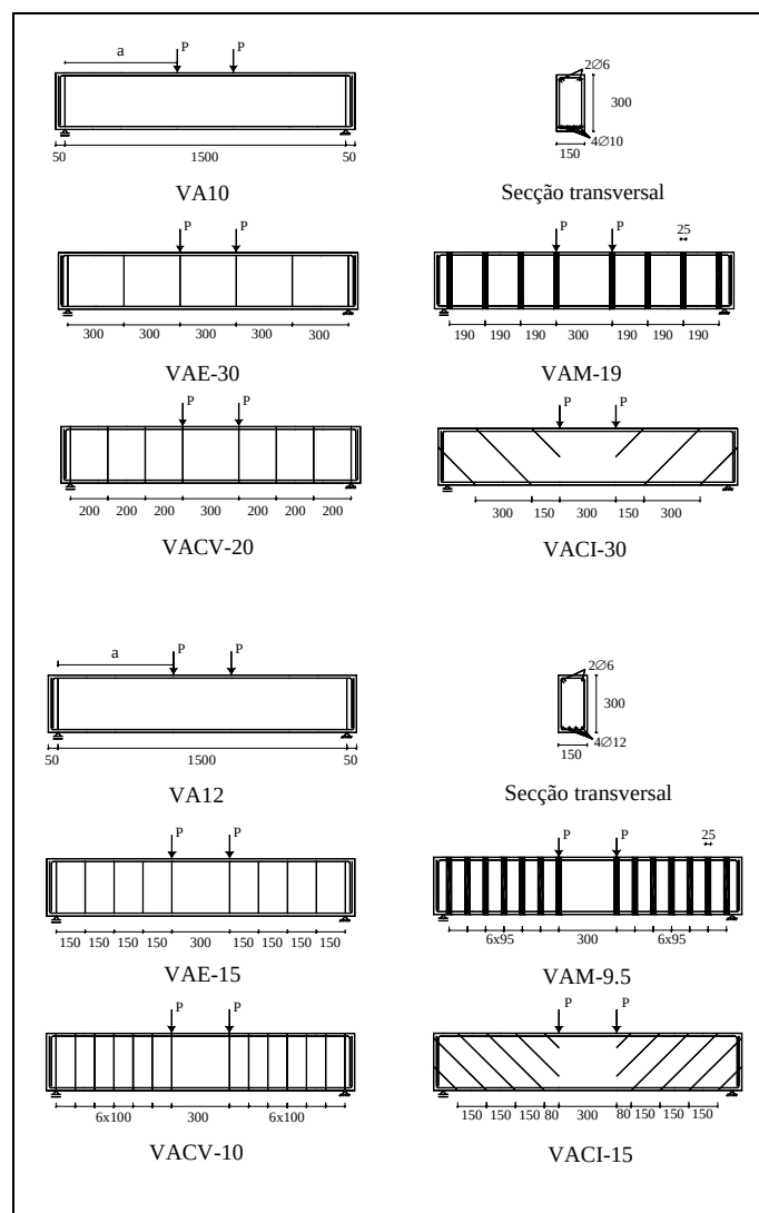
Figura 1 - Características das vigas da série A.
